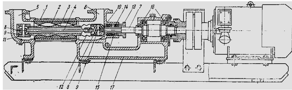
Гвинтовой насос 1Г (1В)
