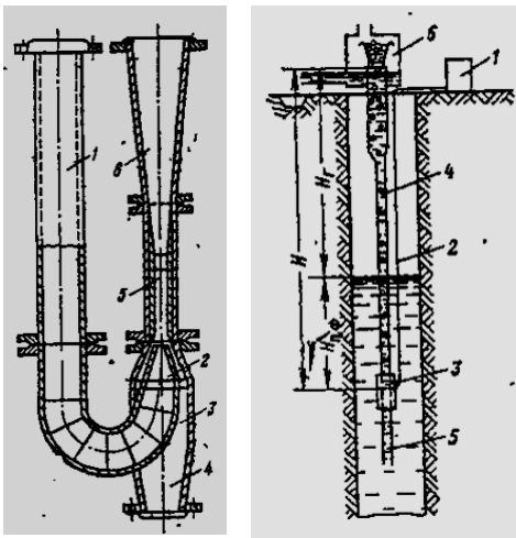
Гідроелеватор
