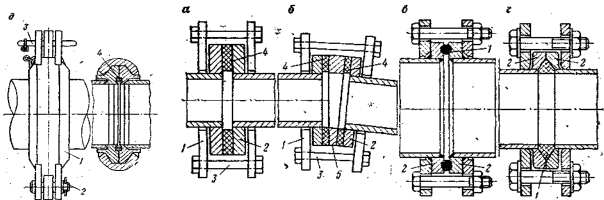
Рис. 72. Фланцеві (а – г) і швидкороз'ємні (д) з'єднання повітропроводів
