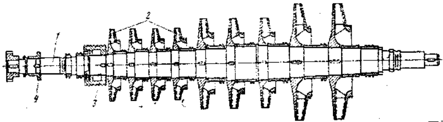
Рис. 67. Ротор відцентрового компресора.
