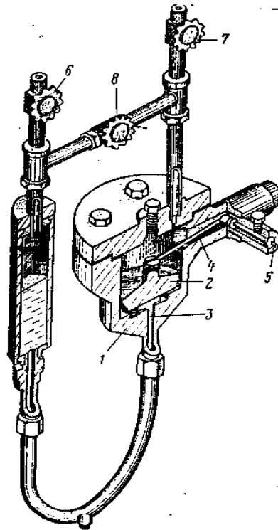
Рис. 70. Дифманометр ДП.
