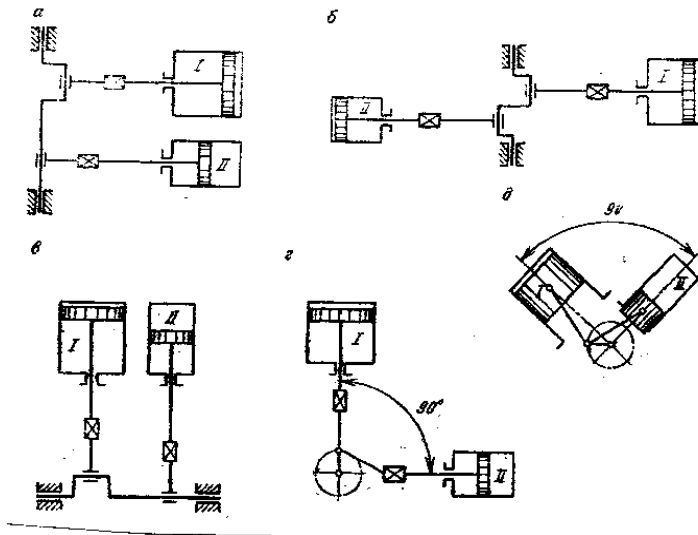
Рис. 61. Двохступеневі поршневі компресори.
