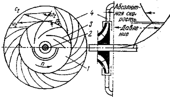
Рис. 66. Ступінь відцентрового компресора
