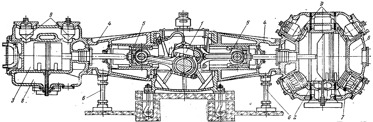
Рис. 62. Компресор 4М10 – 100/8.
