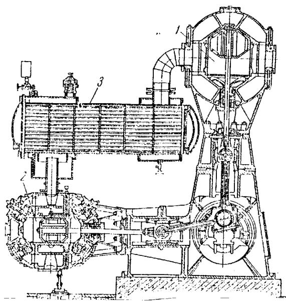
Рис. 63. Компресор ВП – 10/8.
