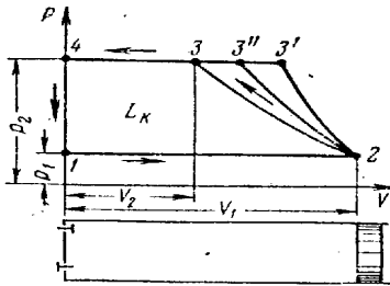
Рис. 57 Діаграма теоретичного процесу в поршневому
