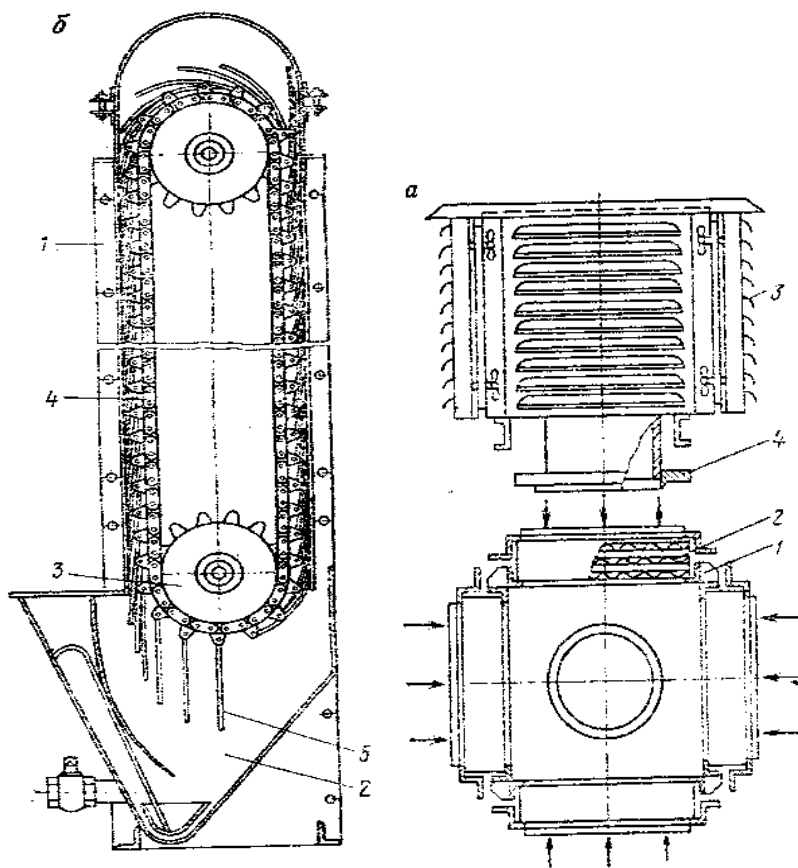
Рис. 71. Фільтри: а – комірковий; б – самоочисний.
