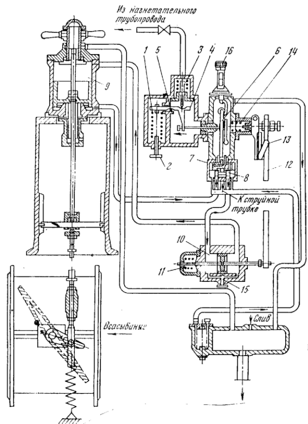
Рис. 69. Регулятор продуктивності відцентрового компресора
