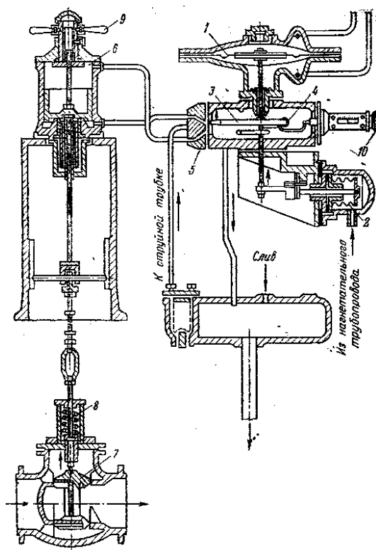
Рис. 68. Протипомпажний захист відцентрового компресора
