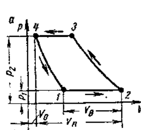
Рис. 58. Діаграма дійсного процесу в
