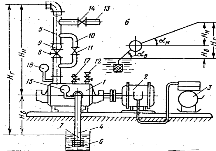
Рис. 39. Водовідливна установка з відцентровим насосом
