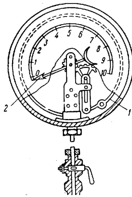
Рис. 54. Манометр.
