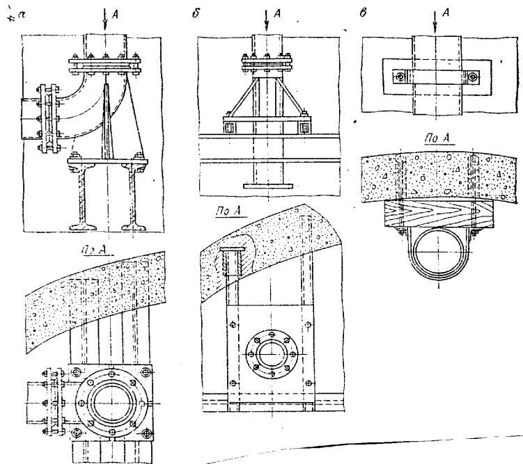
Рис. 53. Пристрої для кріплення труб в стволі: а – опорне коліно, б – опорний стілець, в – хомут.
