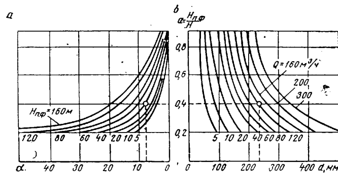
Рис.47. Номограма для розрахунку ерліфта.
