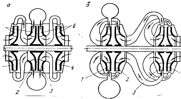
Рис. 42. Симетричне розміщення робочих коліс в насосі
