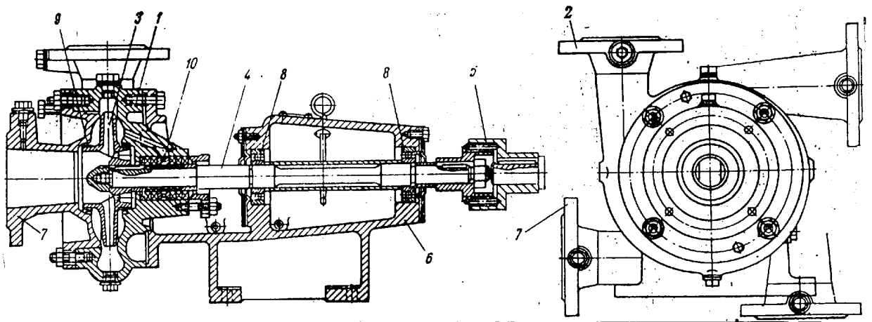
Рис. 43. Консольний насос
