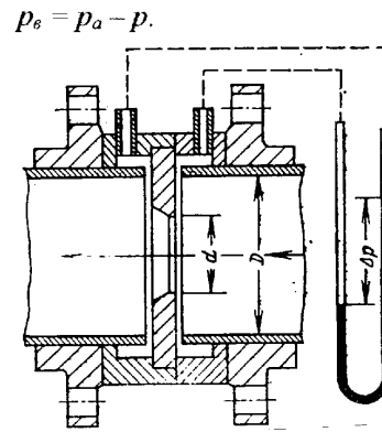
Рис. 55. Дифманометр з діафрагмою.
