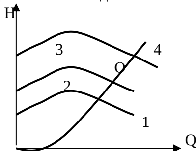
Рис. 49. Діаграма роботи послідовно з'єднаних насосів
