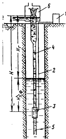
Рис. 46. Ерліфт Гідроелеватор
